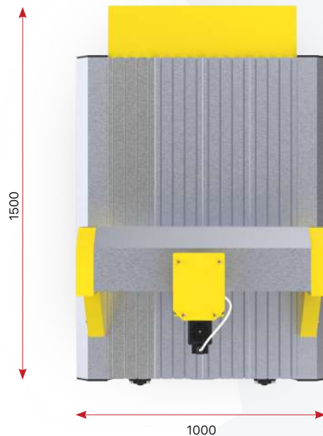
PIANO ORIZZONTALE
